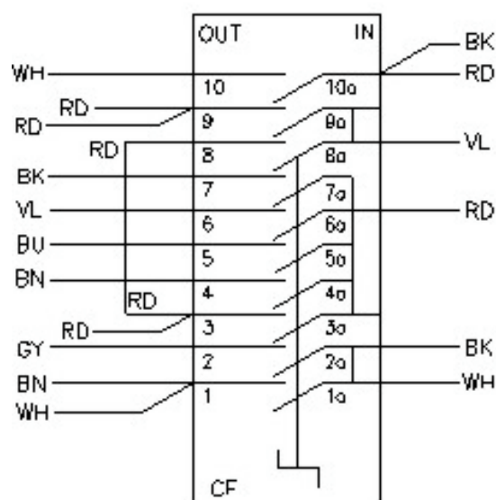
CABLAGGIO 820731339
