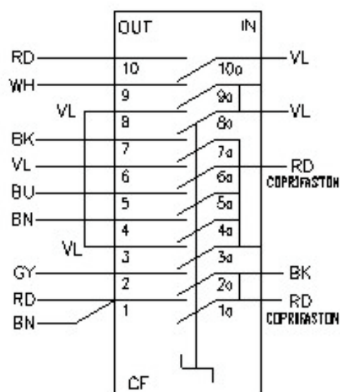
CABLAGGIO 820731354
