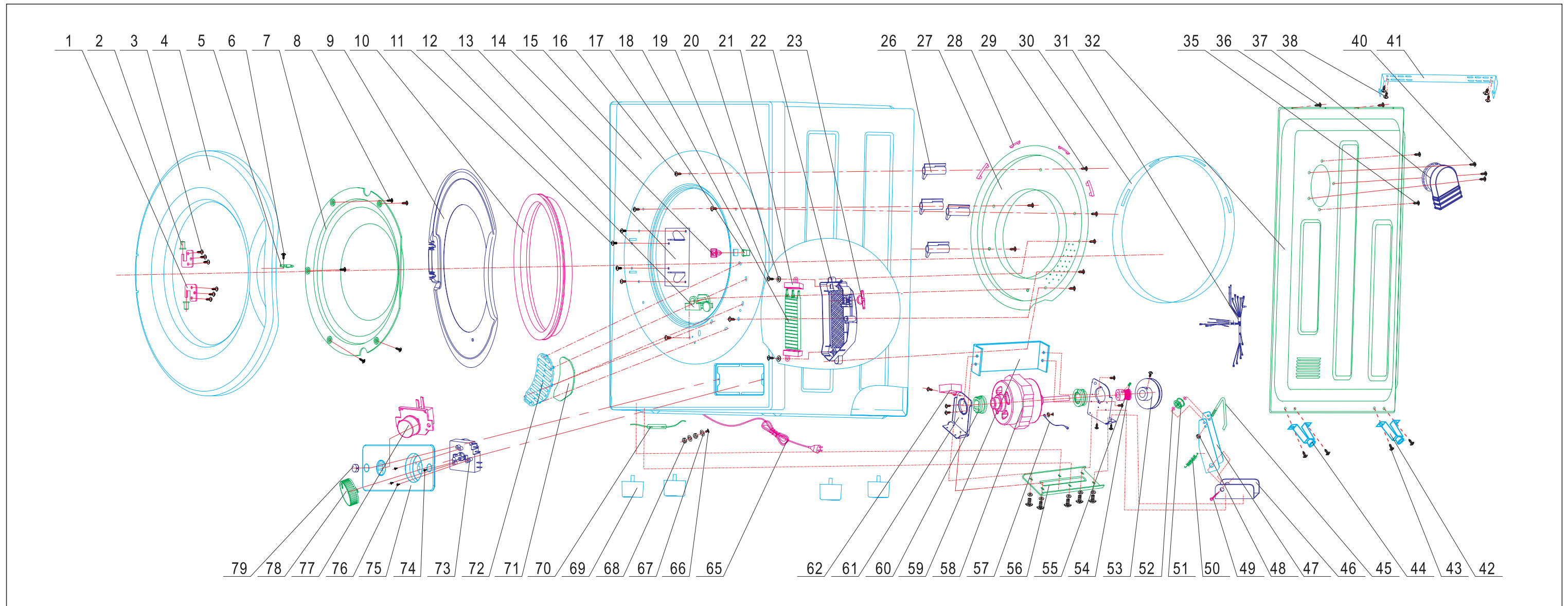
GYJ40-58 爆炸图A
